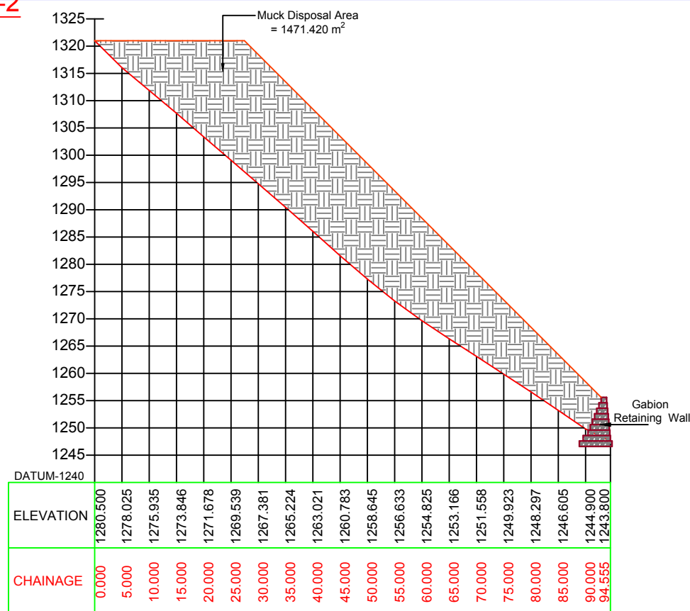
Section At -3 Scale: 1:1000
