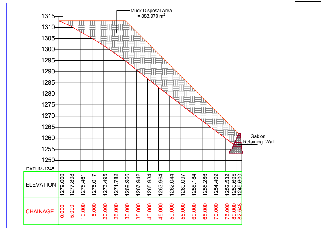
Section At -1 Scale: 1:1000
